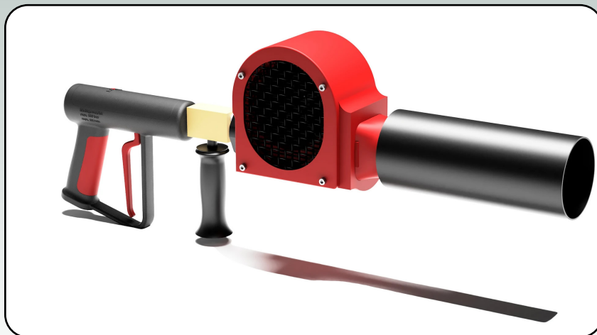
FoamGiant Standard Variante für Löschanlagen mit eingebautem Schaummittelzumischer
